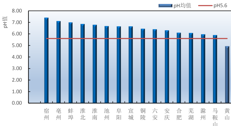
图 5 2021 年 3 月各地级市降水 pH 值
