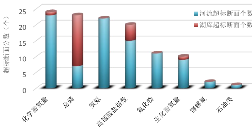
图7 2021年3月全省地表水超标断面主要污染指标
