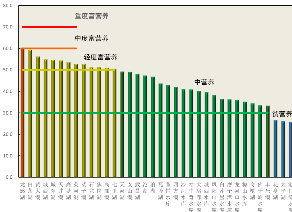
图9 2021年3月主要湖库营养状态指数
