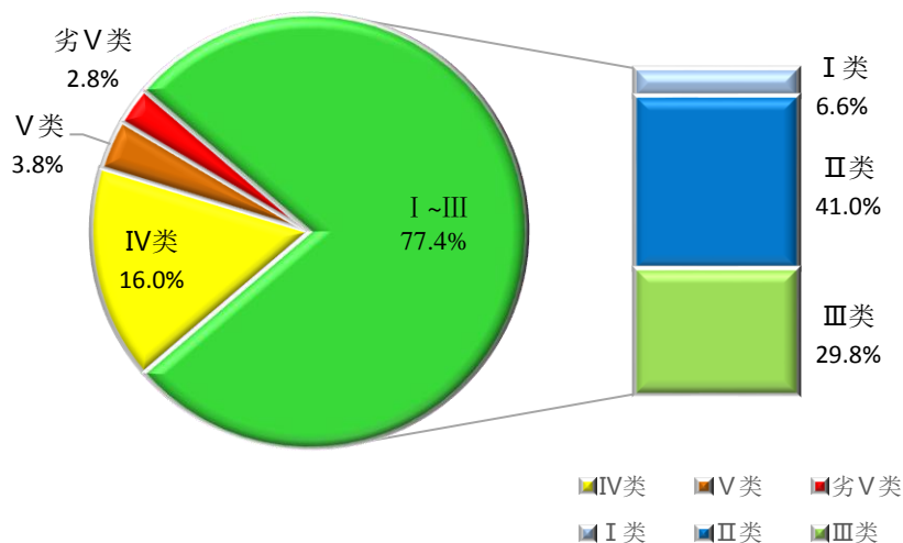
图6 2021年3月全省地表水水质类别比例
