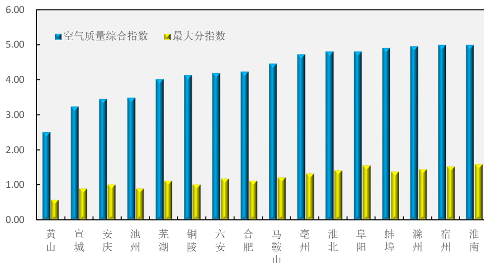
图 4 2021 年 3 月全省各地级市空气质量综合指数
