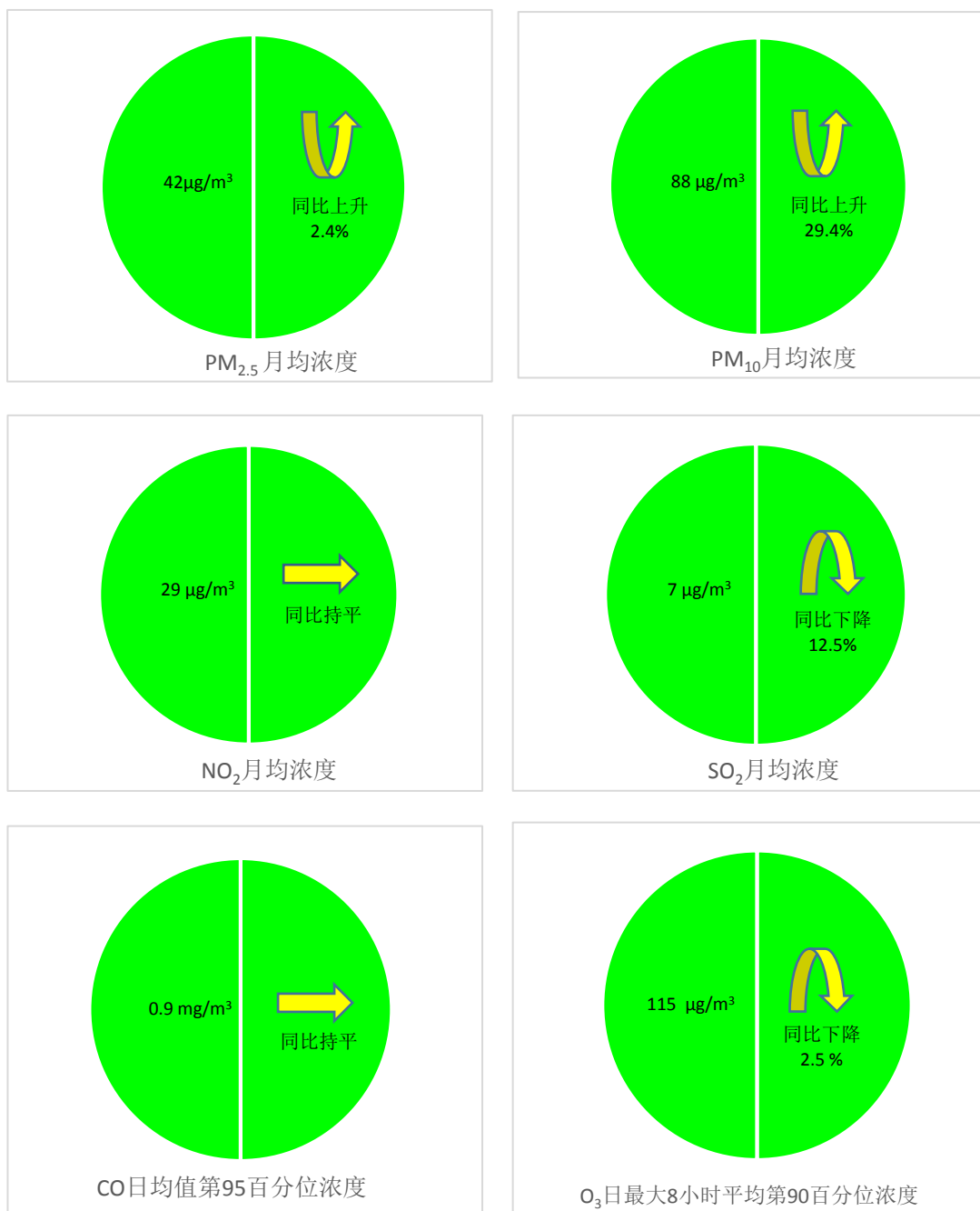
图 3 2021 年 3 月全省主要大气污染物月均浓度
