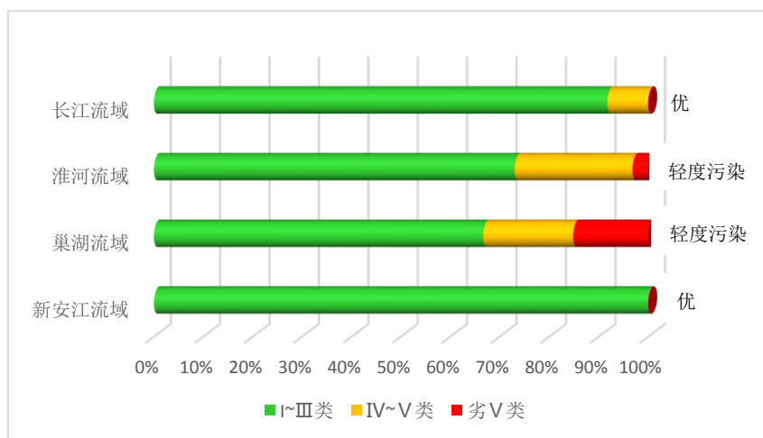
图8 2021年3月全省四大流域水质级别比例
