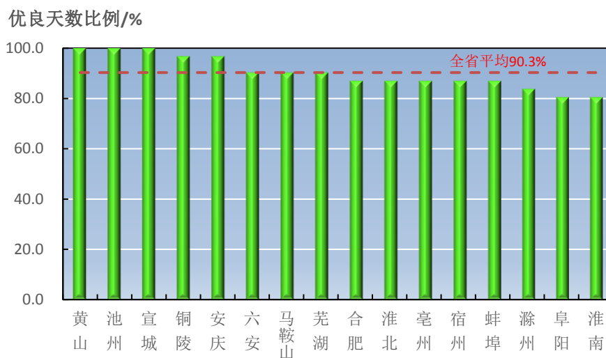
图 2 2021 年 3 月全省各地级市优良天数比例
