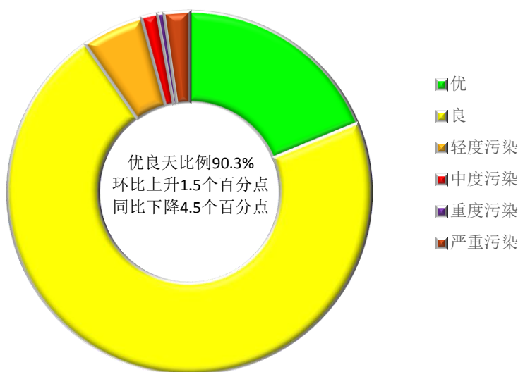
图 1 2021 年 3 月全省平均优良天数比例
